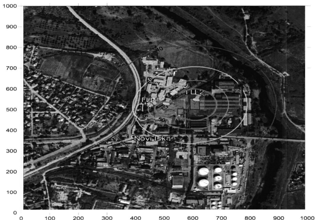
Фигура IV.0-5 Измерителни контури и точки
