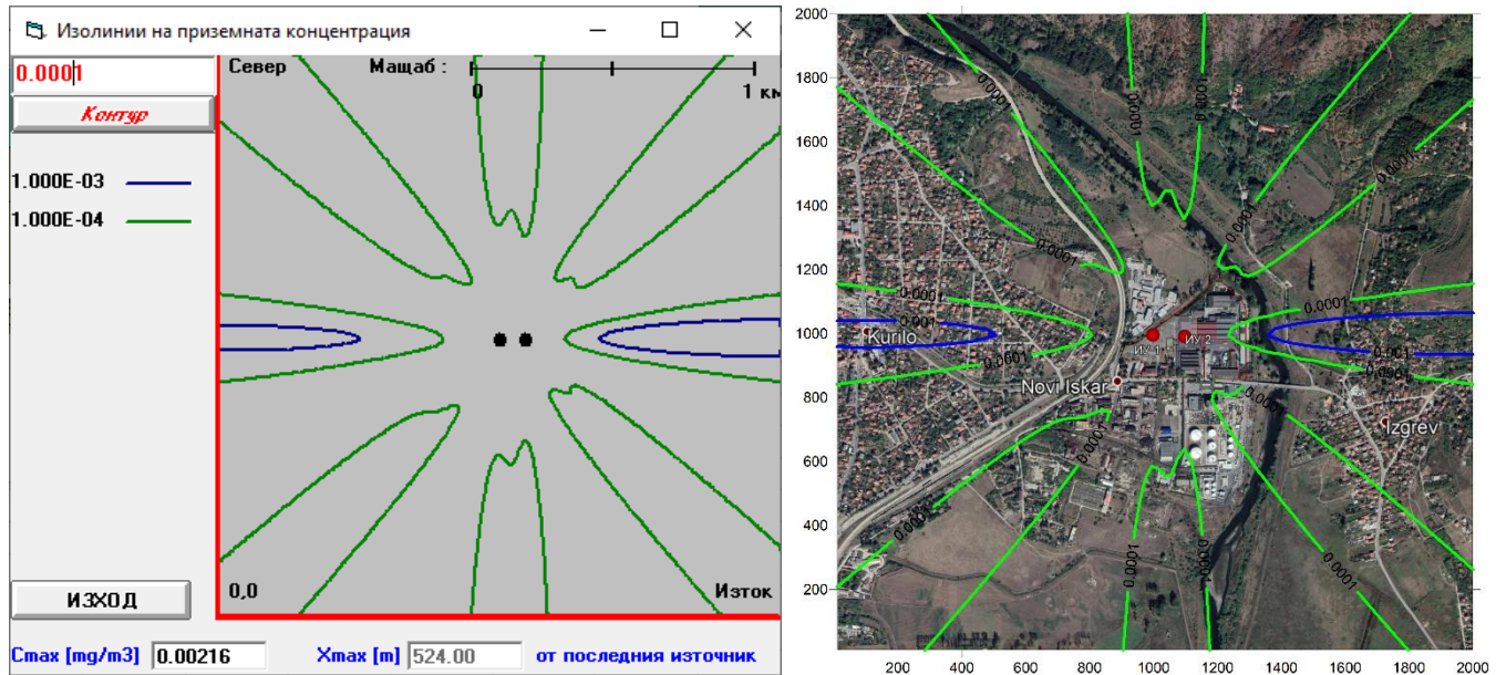
Фигура IV.1.3-3 Изолинии на приземни концентрации на ФПЧ 10 , в съответствие с роза на ветровете
