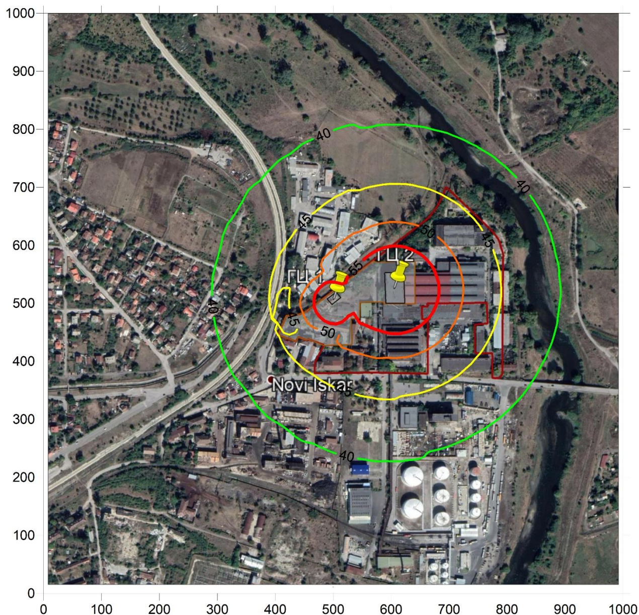
Фигура IV.1-4 Измерителни контури и точки
