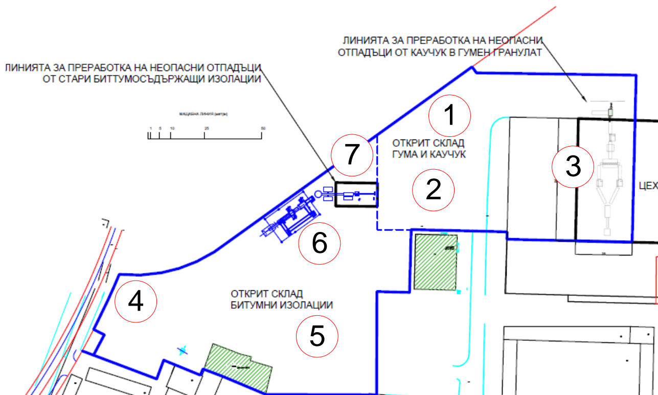
Фигура П.3-1 Генплан на новите производствени линии
