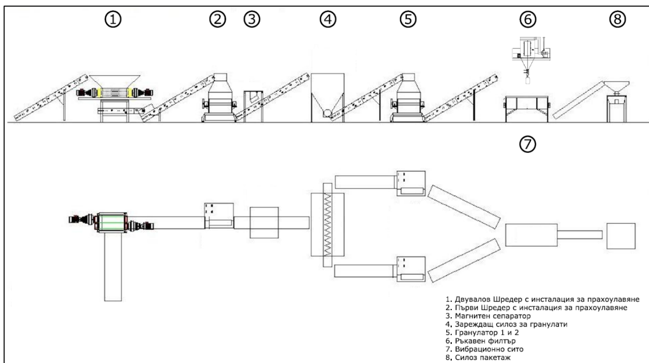
Фигура П.3-2 Технологична схема на линията за третиране на неопасни отпадъци от каучук
