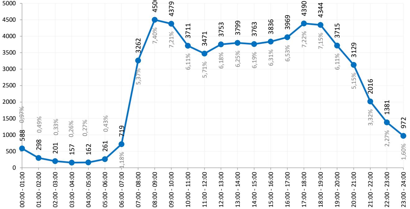
Часова неравномерност за 03.04.2017г на кръстовище бул."П. Яворов" - ул."Стоян Михайловски" КР21 код: 7-53
