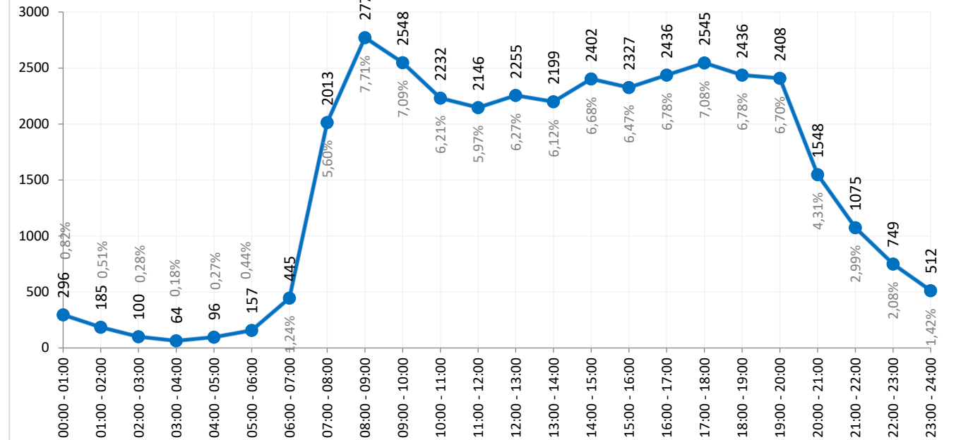
Часова неравномерност за 03.04.2017г на кръстовище бул."Черни връх" - ул."Никола Й. Вапцаров" КР20 код:7-32
