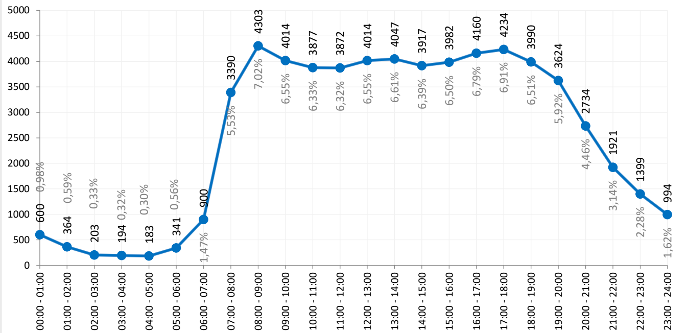
Часова неравномерност за 03.04.2017г на кръстовище бул."Драган Цанков" - бул."Г. М. Димитров" КР23 код:7-58
