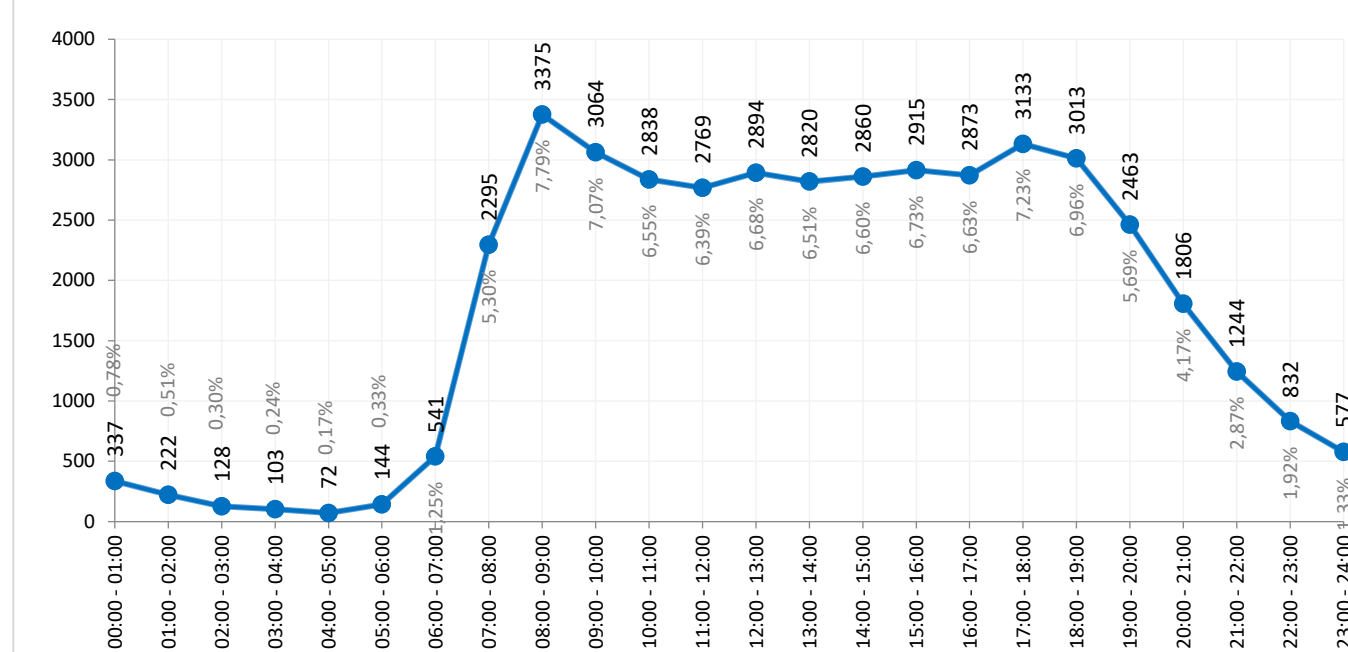
Часова неравномерност за 03.04.2017г на кръстовище бул."Драган Цанков" - ул."Фр. Ж. Кюри" КР 24 код: 7-26
