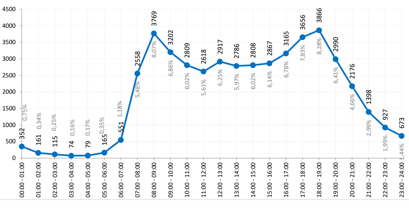
Часова неравномерност за 03.04.2017г на кръстовище бул."Симеоновско шосе" - бул."Г. М. Димитров" КР22 код:7-29
