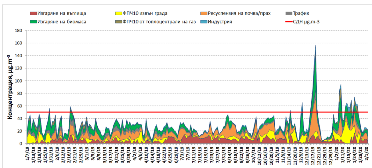
Фиг. 4. Времеви годишен ход на приноса на различните източници на ФПЧ 10
