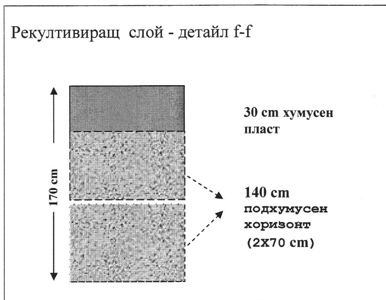
Фигура 4. Схема на рекултивиращ слой с дебелина 170cm
