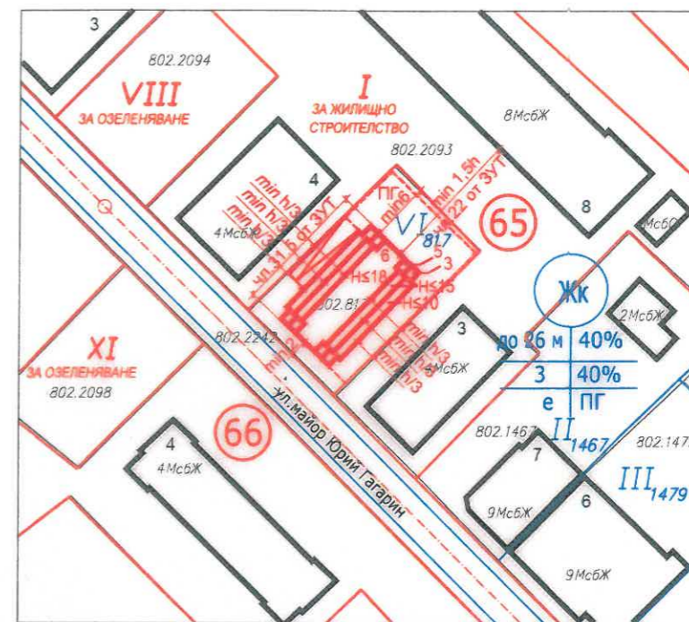
Изменение на План за застрояване за УПИ VI-817, кв. 65, м. "Изток - Изток" - Част 1 и Част 2, р-н Изгрев СО М 1:1000
