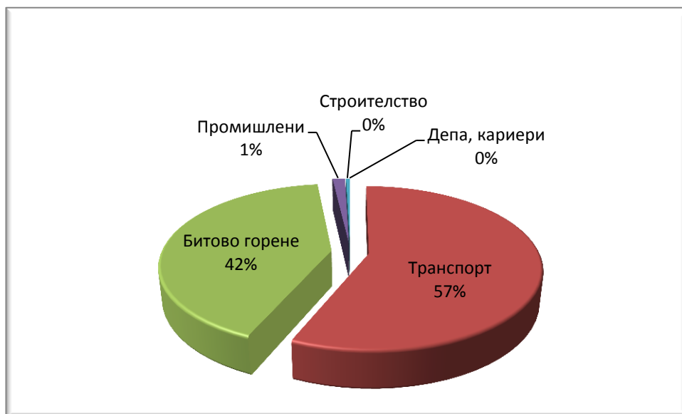
Фигура 5.5 Принос на отделните сектори към общата емисия, t/y , на \text{ФПЧ}_{10} за 2014 г.
