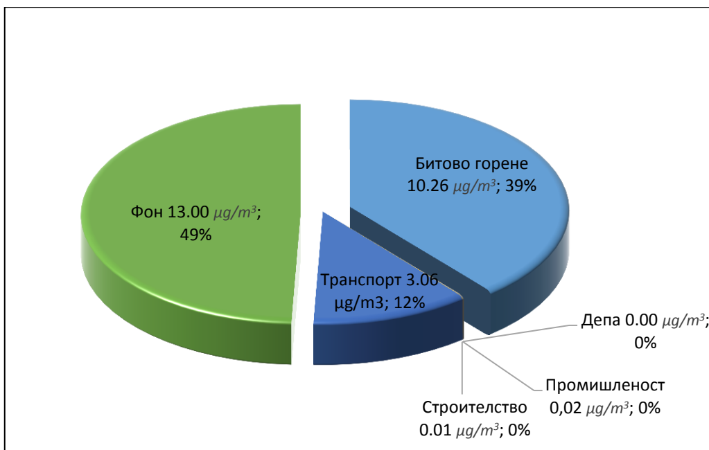
Фигура 6.7 Относителен принос на отделните групи източници към СГК на ФПЧ 10 в ПМ Гара Яна за 2014 г.
