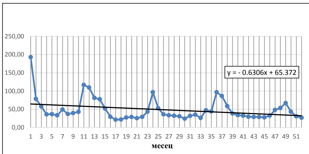
Фигура 4.21 Средномесечна концентрация на ФПЧ 10 , \mu\text{g}/\text{m}^3 , пункт Надежда
