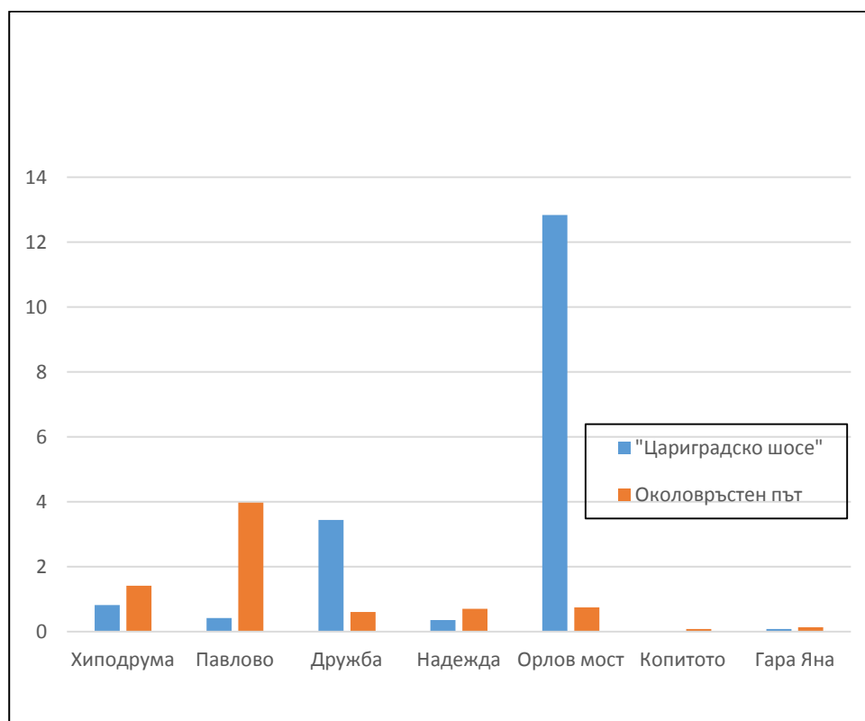
Фигура 6.23 СГК на ФПЧ 10 , \mu\text{g}/\text{m}^3 , обусловена от трафика по южна дъга на Околовръстен път и "Цариградско шосе"
