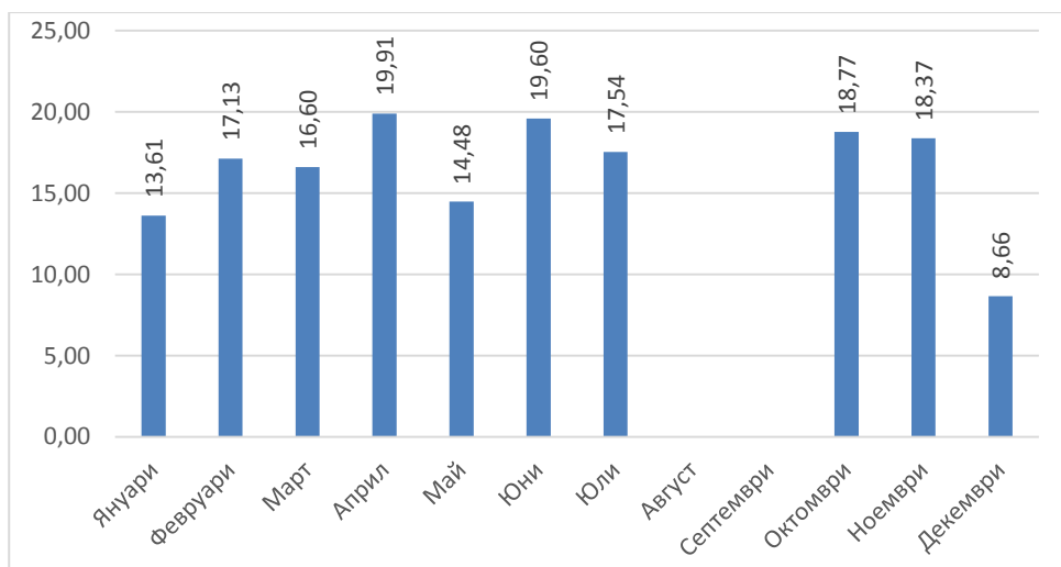
Фигура 4.47. Средномесечни стойности на концентрацията на \text{ФПЧ}_{10} за 2014 г. в мониторингов пункт „Копитото“, \mu\text{g}/\text{m}^3
