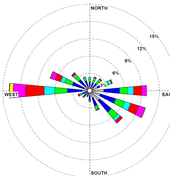
Роза на вятъра за 2009 г. Тихо време 23.07 %
