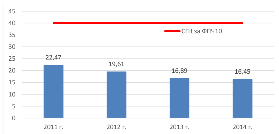
Фигура 4.43 Средногодишна концентрация на ФПЧ 10 в пункт Копитото за периода 2011-2014 г.
