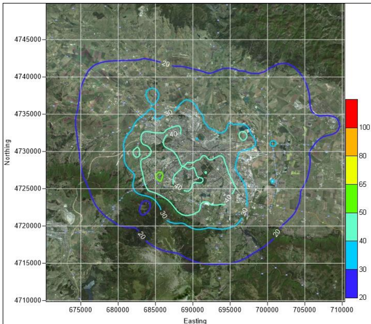
Фигура 8.14 Стойности на 90.4-тия перцентил на СДК на \text{ФПЧ}_{10} , \mu\text{g}/\text{m}^3 , от всички източници и фон за 2020 година
