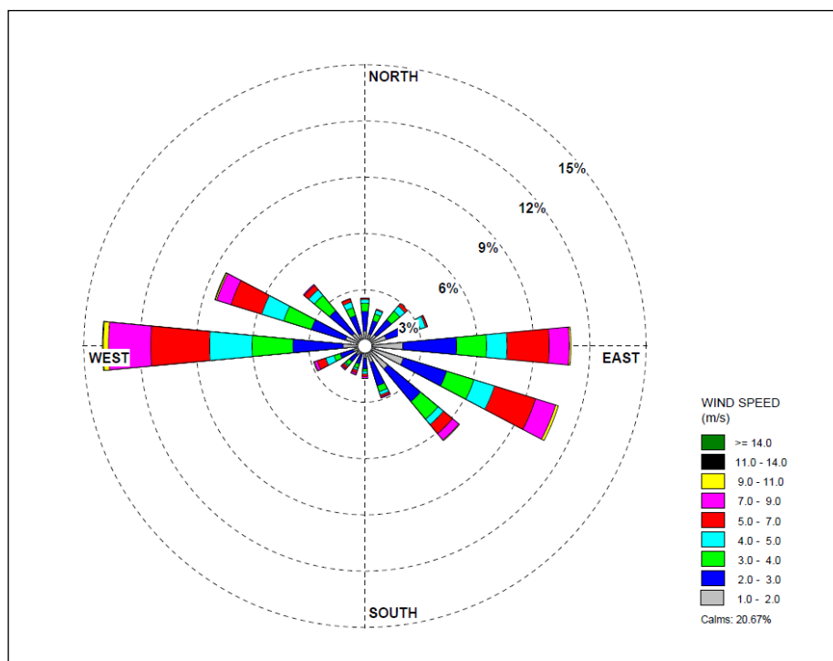
Фигура 2.7 Роза на вятъра за станция София – 2010 г.
