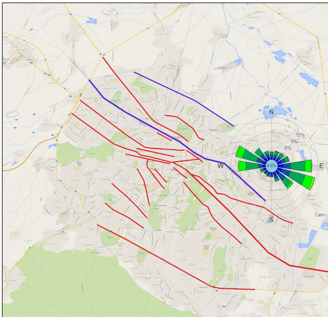
Фигура 6.35 Ориентация на основни транспортни артерии с интензивен трафик, в София спрямо розата на вятъра за 2014 година
