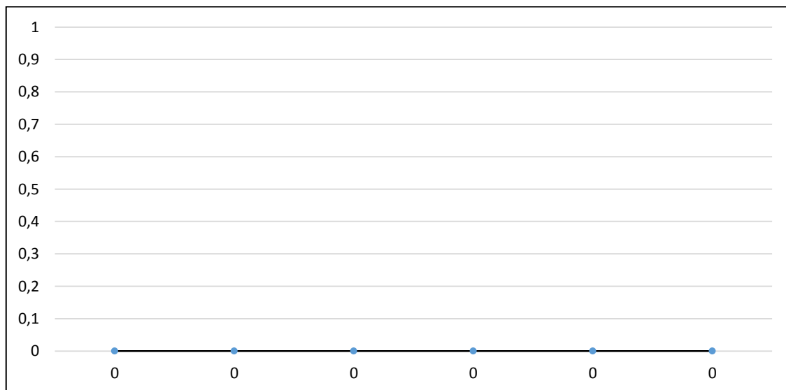
Фигура 5.10 Измерена средногодишна концентрация на \text{ФПЧ}_{10} , \mu\text{g}/\text{m}^3 , в пункт за мониторинг Копитото, за периода 2009 – 2014 година
