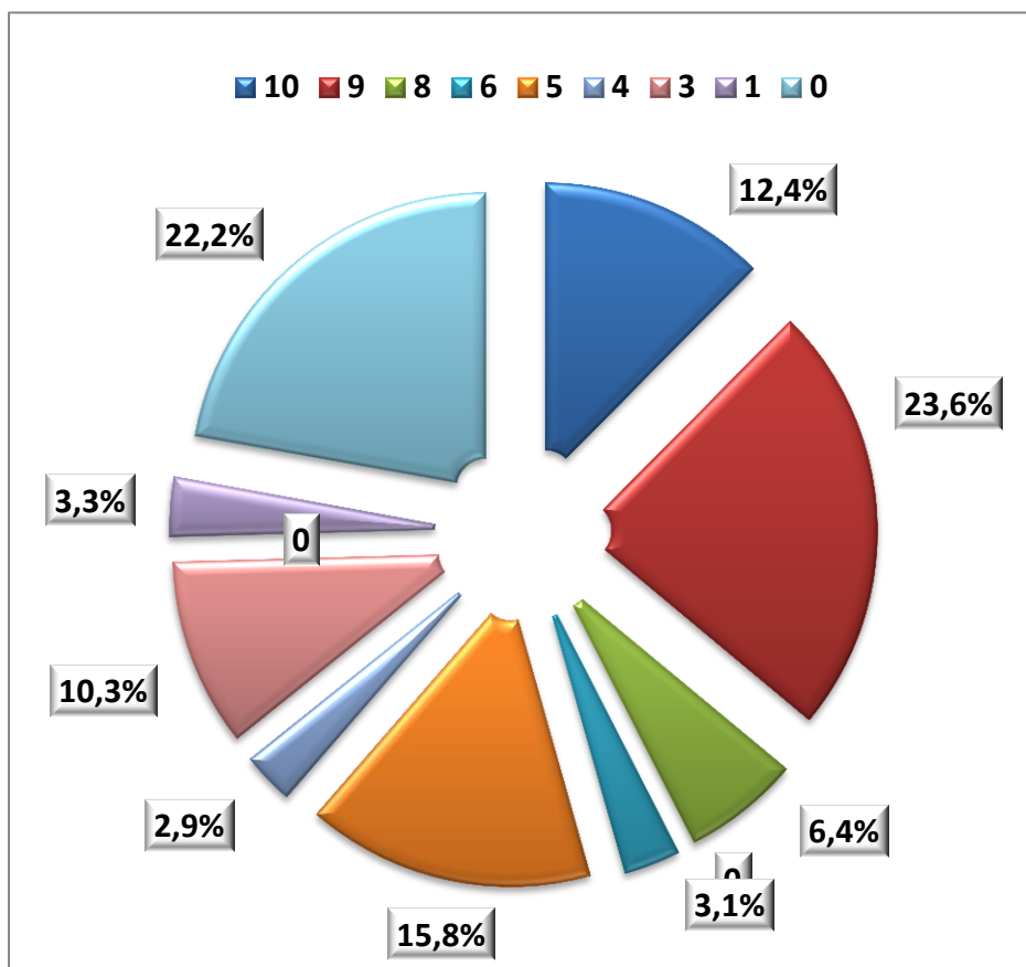
Фигура 6.32 Облачност през 2009 г.
