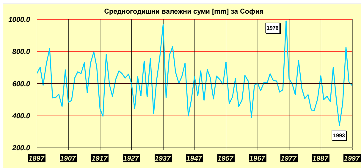
Фигура 2.9 Валежи в София за 100 годишен период.
