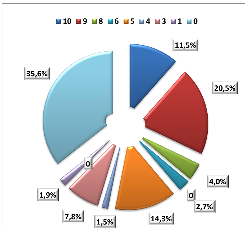
Фигура 6.31 Облачност през 2008 г.
