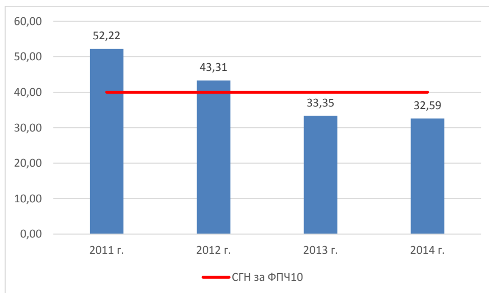
Фигура 4.1 Средногодишна концентрация на \text{ФПЧ}_{10} в Гара Яна за периода 2011 – 2014г.
