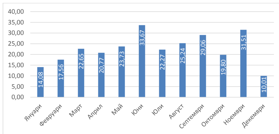
Фигура 4.44 Средномесечни стойности на концентрацията на \text{ФПЧ}_{10} за 2011 г. в мониторингов пункт „Копитото“, \mu\text{g}/\text{m}^3
