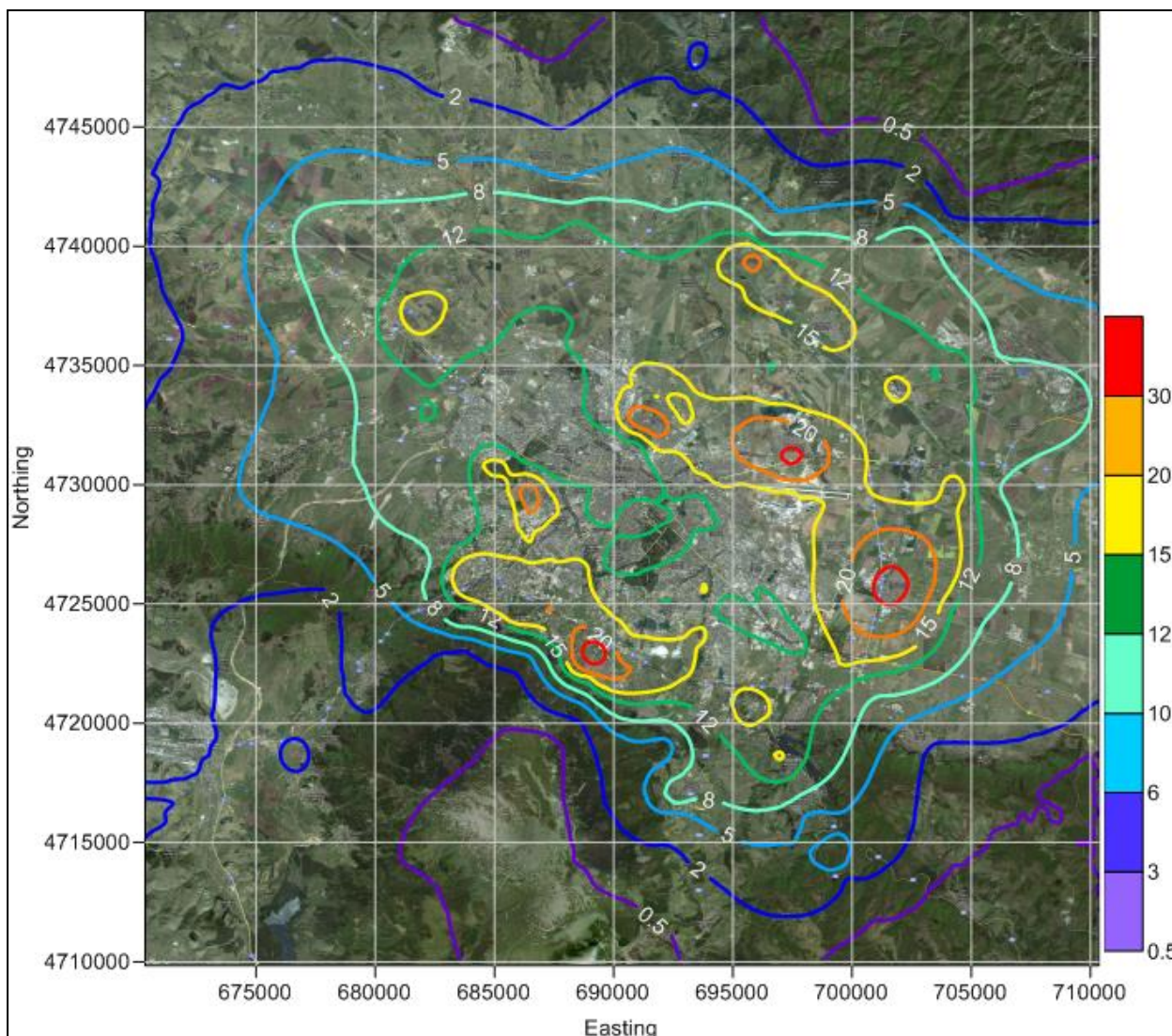
Фигура 6.6 СГК на ФПЧ 10 , \mu\text{g}/\text{m}^3 , обусловена от битово горене за 2014 година
