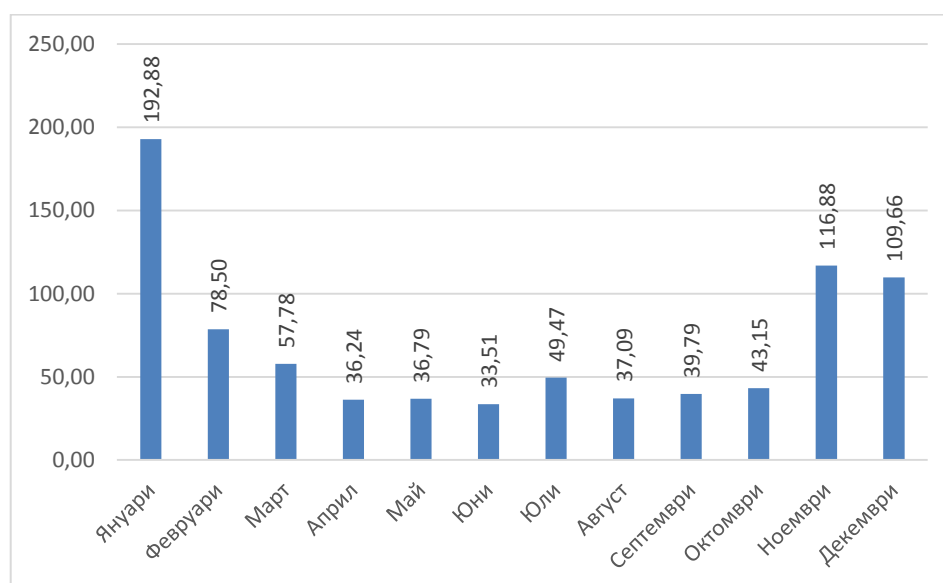
Фигура 4.16 Средномесечна концентрация на \text{ФПЧ}_{10} за 2011 г. в пункт Надежда
