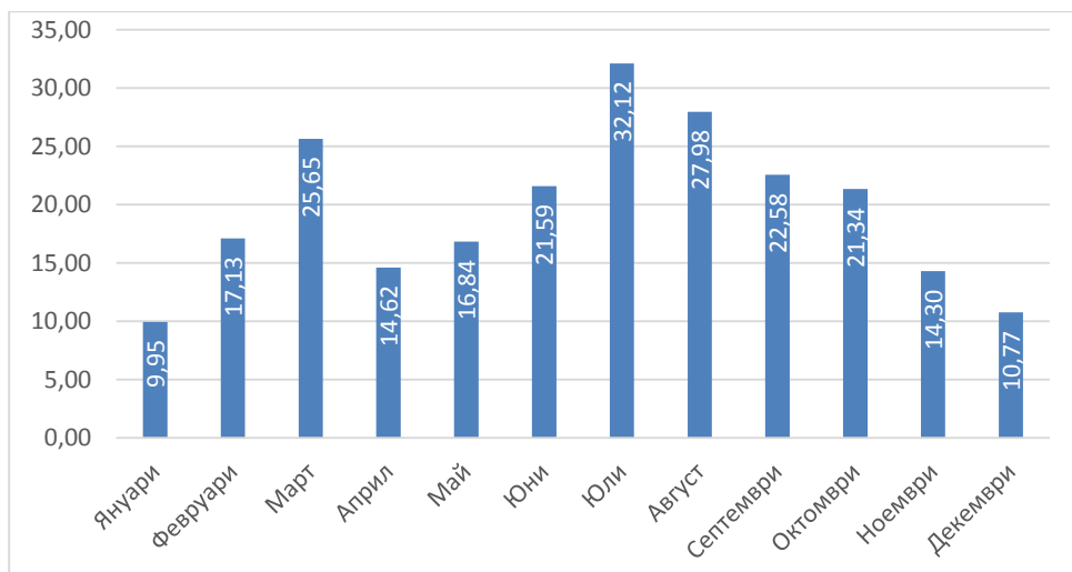
Фигура 4.45. Средномесечни стойности на концентрацията на \text{ФПЧ}_{10} за 2012 г. в мониторингов пункт „Копитото“, \mu\text{g}/\text{m}^3
