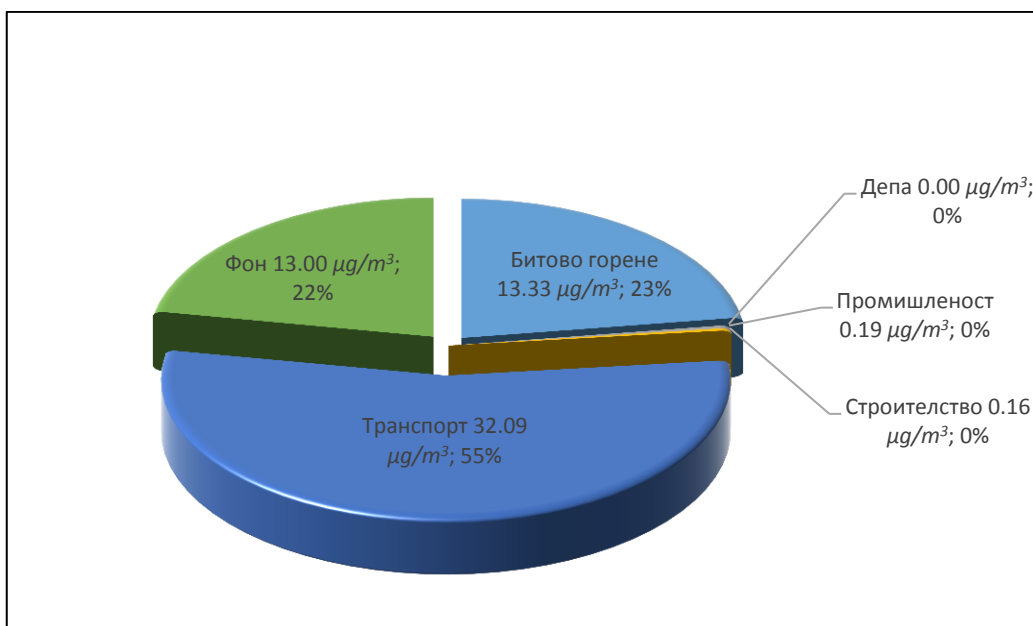
Фигура 6.8 Относителен принос на отделните групи източници към СГК на ФПЧ 10 в ПМ Орлов мост за 2014 г.
