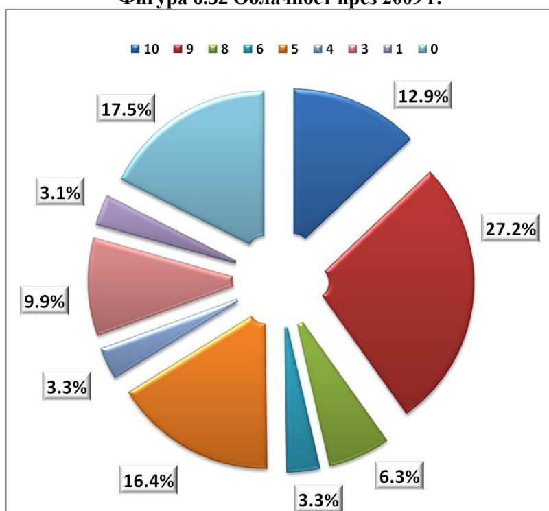
Фигура 6.33 Облачност през 2010 г.
