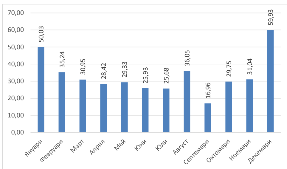
Фигура 4.3 Средномесечна концентрация на ФПЧ 10 за 2012 г. в пункт Гара Яна
