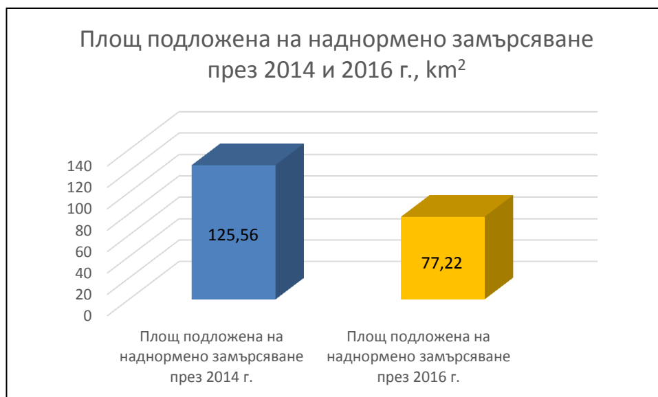
Фигура 8.10 Площи от територията на Столична община, подложени на наднормено замърсяване с ФПЧ 10 за 2014 и 2016 г.
