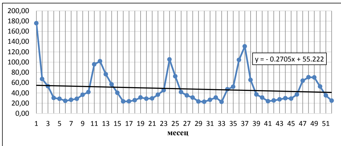
Фигура 4.42 Средномесечна концентрация на ФПЧ 10 , \mu\text{g}/\text{m}^3 , пункт Павлово за периода 2011- април 2015 г.
