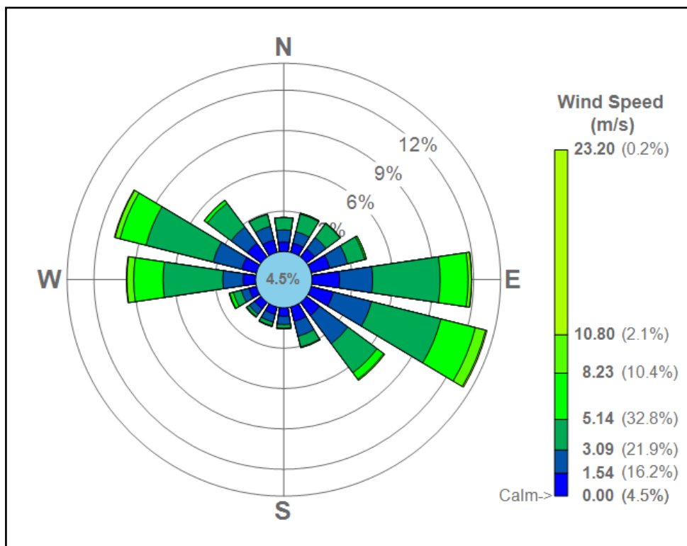
Фигура 6.2 Роза на вятъра за станция София – 2014 г.
