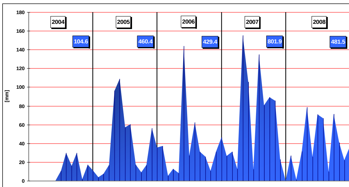
Фигура 2.10 Валежи в София за пет години.
