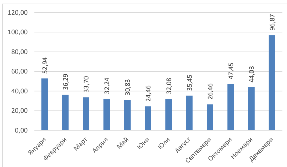
Фигура 4.18 Средномесечна концентрация на ФПЧ 10 за 2013 г. в пункт Надежда
