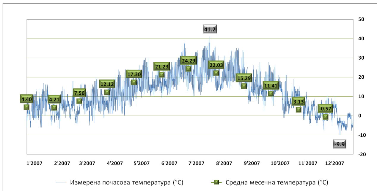
Фигура 6.26 Температура за 2007 г.
