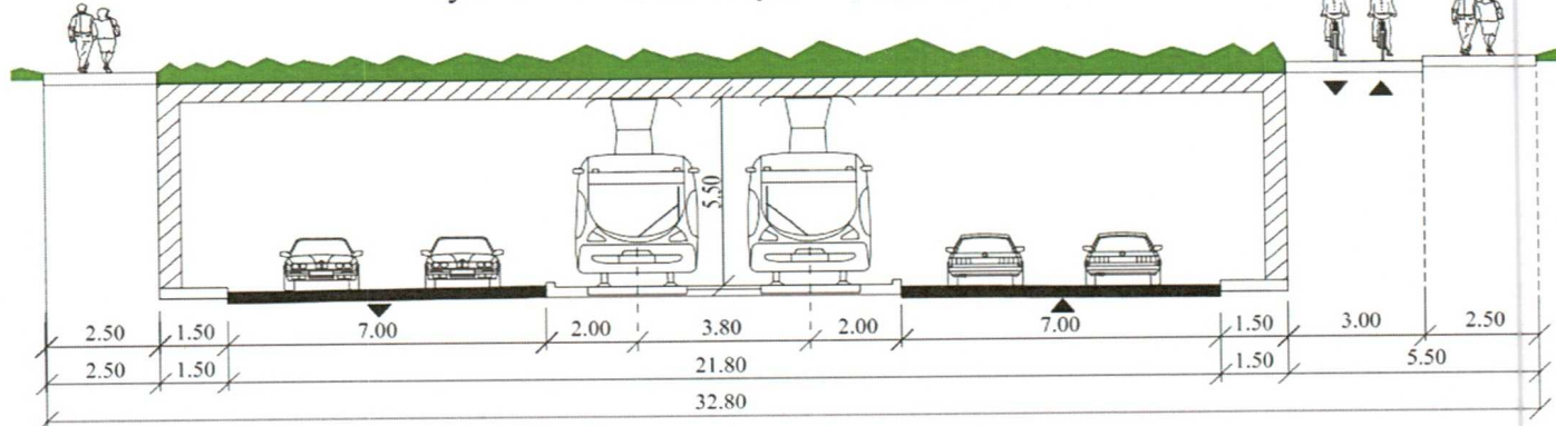
бул. "Монтевидео" в тунел разрез 6-6
