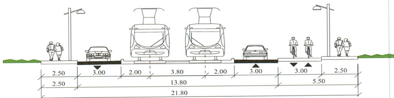
бул. "Монтевидео" разрез 5-5
