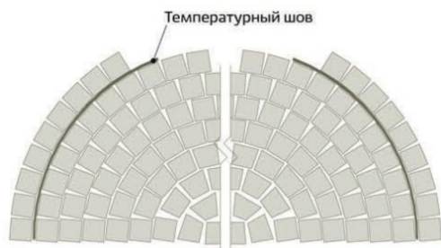
Тип 8. Радиальная кладка Используемая плитка — брусчатка
