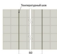
Тип 3. Штабельная перевязка Используемая плитка — квадратная
