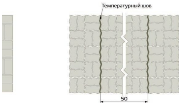
Тип 6. Кладка узором «плетенка» Используемая плитка — фигурная тротуарная
