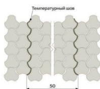
Тип 7. Комбинированный шестиугольник Используемая плитка — фигурная тротуарная
