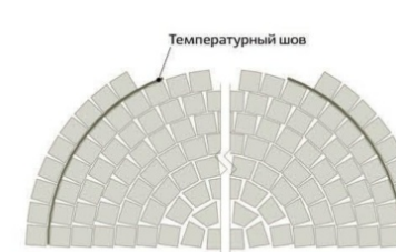
Тип 8. Радиальная кладка Используемая плитка — брусчатка
