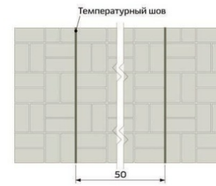
Тип 5. Кладка узором «плетенка» Используемая плитка — прямоугольная тротуарная
