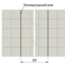
Тип 3. Штабельная перевязка Используемая плитка — квадратная
