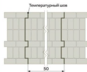
Тип 4. Смешанная ложковая и штабельная перевязка Используемая плитка — прямоугольная
