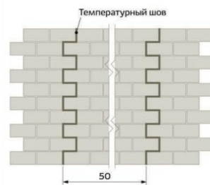
Тип 1. Ложковая перевязка Используемая плитка — прямоугольная
