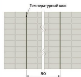
Тип 2. Штабельная перевязка Используемая плитка — прямоугольная
