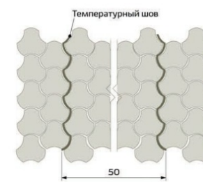
Тип 7. Комбинированный шестиугольник Используемая плитка — фигурная тротуарная
