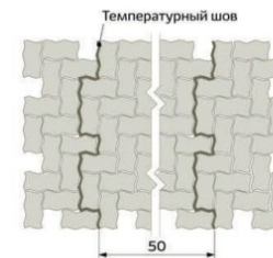
Тип 9. Перевязка «в елку» Используемая плитка — фигурная тротуарная
